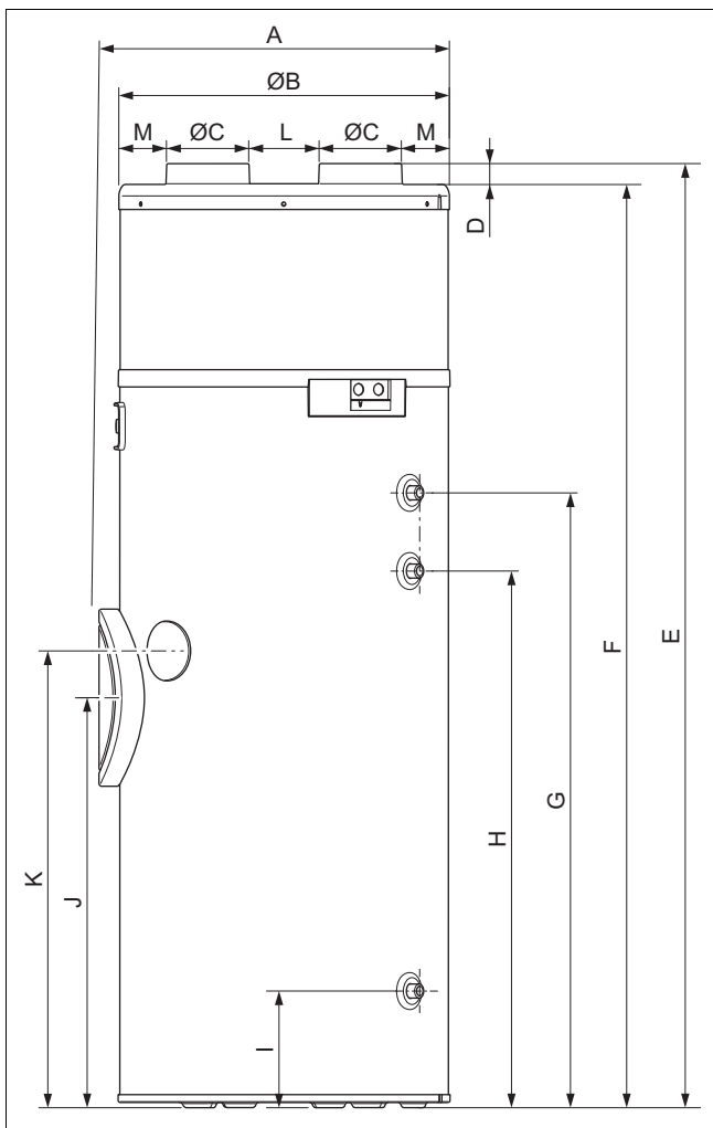
Dimensions de l'appareil et cotes de raccordement
